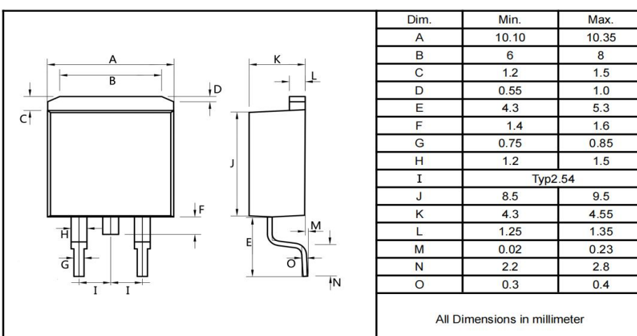
TO-263
